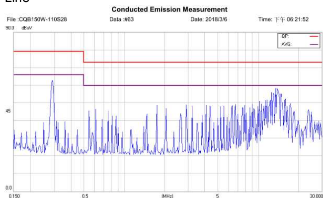
CQB150W-110S28-CMFC(D) Line
