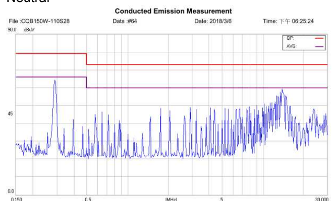
CQB150W-110S28-CMFC(D) Neutral
