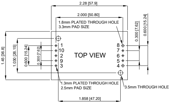
Option Module
